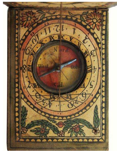
Nürnberg Klappsonnenuhr mit Deklinationskorrektur des „Kompastensmachers“ Kleininger Mitte 19. Jahrhundert
